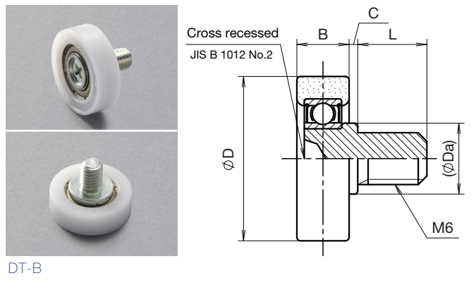
モデル 4 ねじ軸タイプ（十字穴付）
