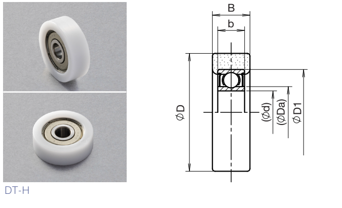
モデル 1 貫通穴タイプ（インナーレース幅凹）
