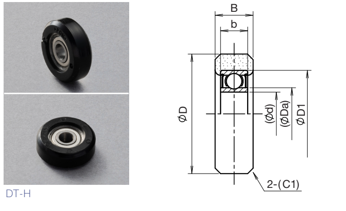
モデル 2 貫通穴タイプ（インナーレース幅凹・アウターレースC面取り付）
