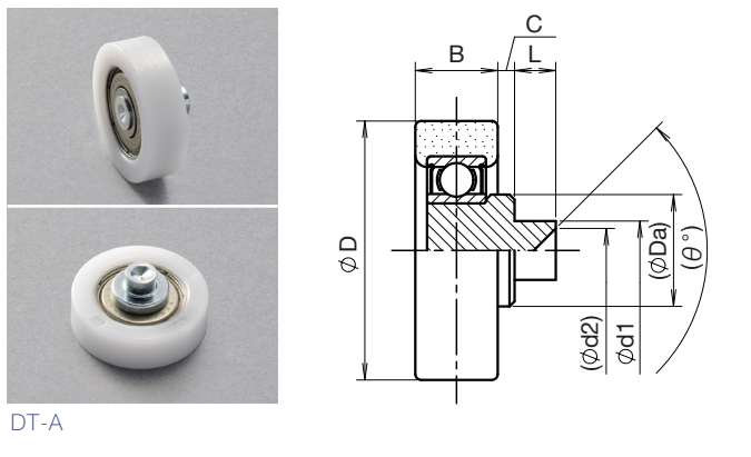
モデル 3 カシメ軸タイプ
