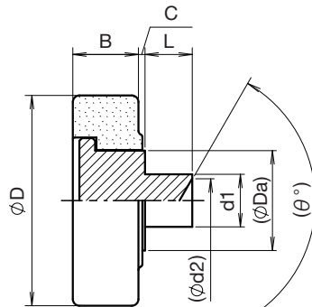
モデル 2 カシメ軸タイプ
