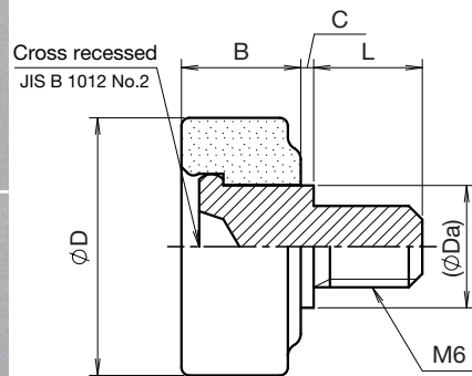
モデル 3 ねじ軸タイプ（十字穴付）
