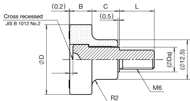
モデル 4 ねじ軸タイプ（十字穴付き・長尺サイズ）
