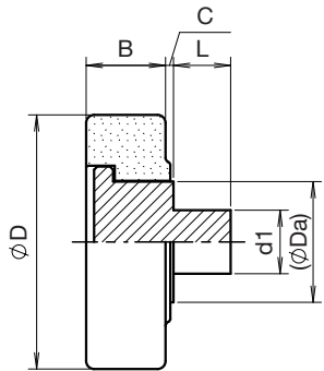
モデル 1 カシメ軸タイプ（ザグリなし）
